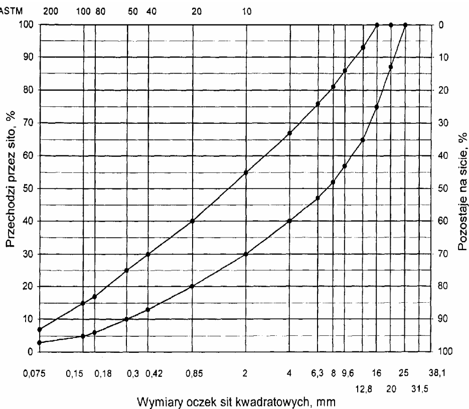
Rys. 8. Krzywe graniczne uziarnienia mieszanki mineralnej BA od 0 do 20 mm do warstwy wiążącej, wyrównawczej i wzmacniającej nawierzchni drogi o obciążeniu ruchem KR1 lub KR2
